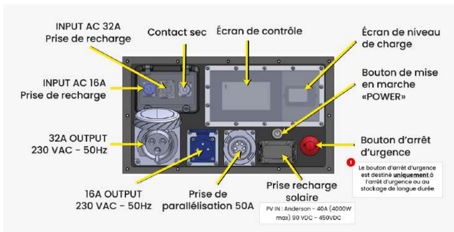
Figure 1: Face arrière de l'appareil
